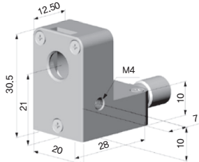
TM-APL-CS 에어 퍼지 칼라, 라미나형
