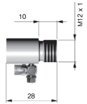
TM-AP-CS 10:1 센서용 에어 퍼지 칼라
