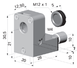
TM-APLCF-CS 에어 퍼지 칼라, 라미나형, 내장형 CF 렌즈
