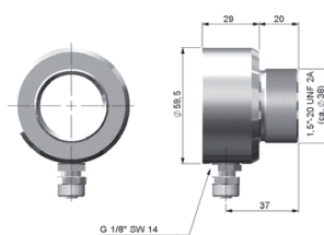
TM-AP-CX CX 센서용 에어 퍼지 칼라
