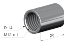
TM-PA-CT 반사 방지 튜브용 파이프 어댑터
