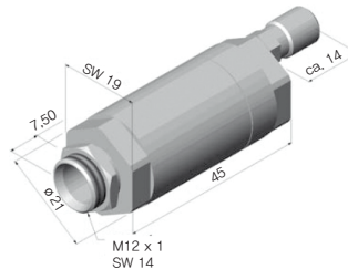
TM-AP-CT 10 : 1 / 15 : 1 / 22 : 1 렌즈용 표준 에어 퍼지 칼라 TM-APS-CT 에어 퍼지 칼라, 스테인리스 스틸
