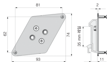
TM-RAIL-CT 컨트롤러용 레일 마운트 어댑터
