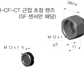
TM-CFAG-CT CF 렌즈 수나사 TM-PWAG-CT 보호 윈도우용 수나사
