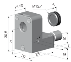
TM-APLCF-CT CF 렌즈 / 보호용 윈도우 · 에어 퍼지 칼라용 내장 옵션
