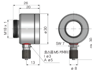
TM-APMH-CT 대형 하우징용 에어 퍼지 칼라, 스테인리스 스틸
