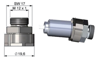
TM-TAS-CT CT 센서용 피벗 조인트
