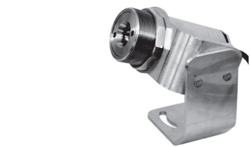
마운팅 브라켓 (TM-AB-CTL)에 설치되는 수냉식 하우징 (TM-W-CTL) 및 에어 퍼지 칼라 (TM-AP-CTL)
