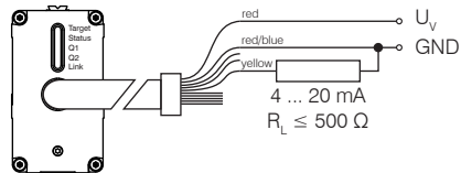
Fig. 11 Wiring analog output
