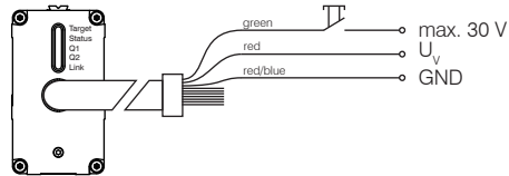
Fig. 17 Wiring trigger input
