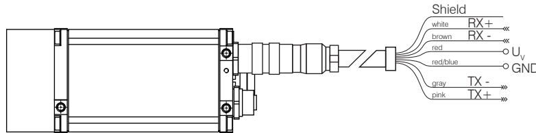
Fig. 14 Wiring RS422
