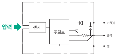
내부 회로도
