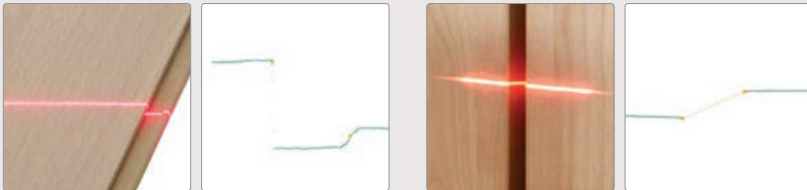
파케이 마룻장 엷지의 프로파일 검사
